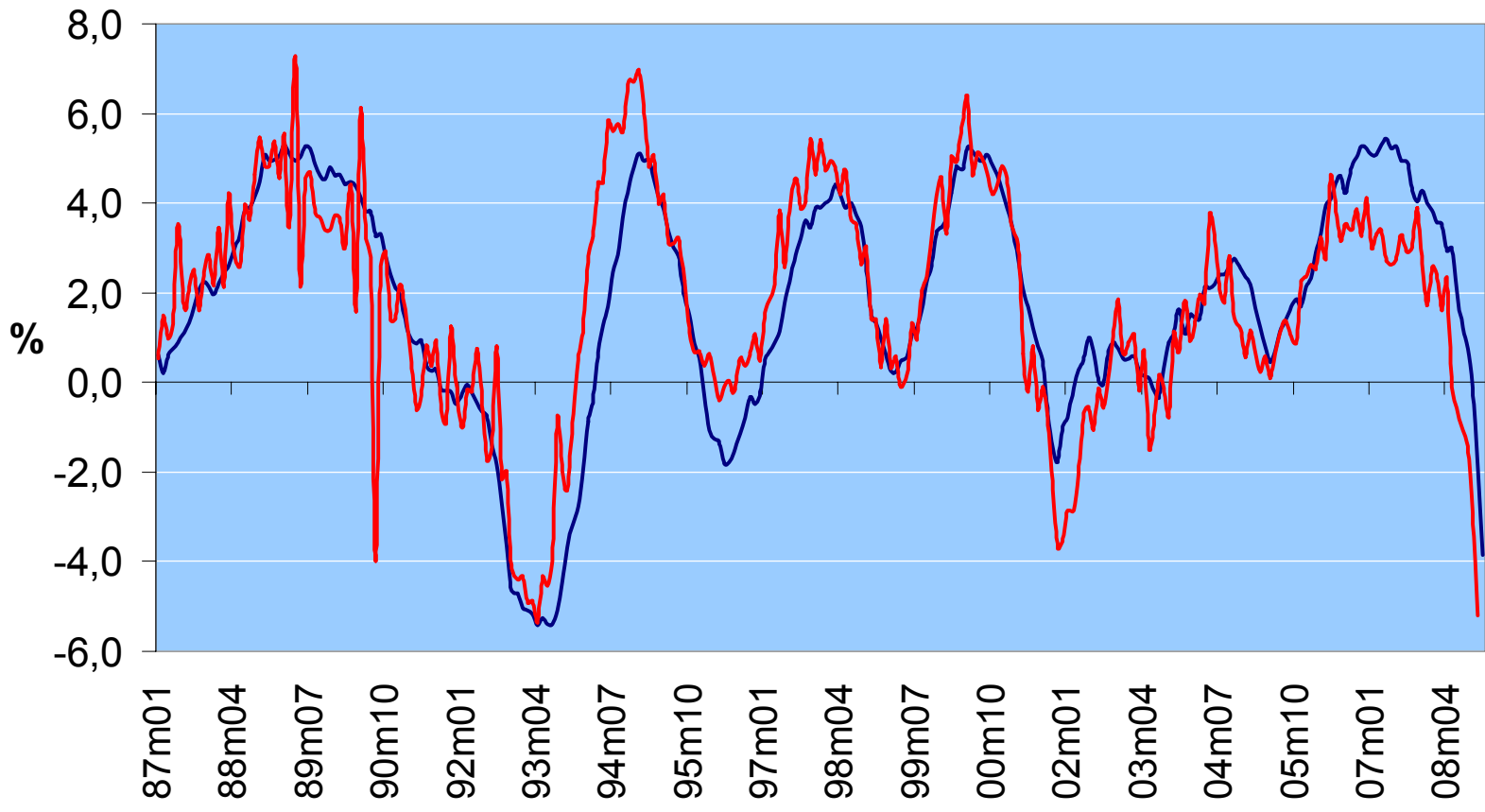
— Geschäftsklimaindex — Industrieproduktion
